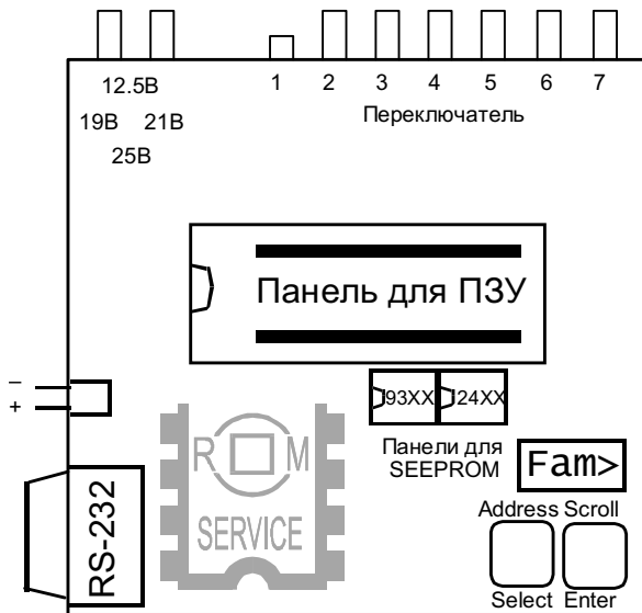
Рис. 1 Внешний вид программатора МП-9М и расположение клавиш.
