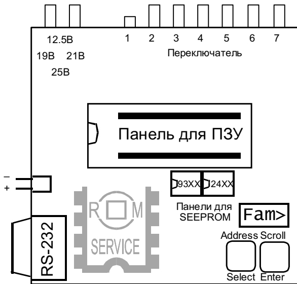
Рис. 1 Внешний вид программатора МП-11 и расположение клавиш.
